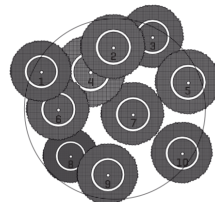
BOTTOM VIEW | VISTA INFERIOR POSITION LAMP SHADES | POSICIÓN DE LAS TULIPAS
